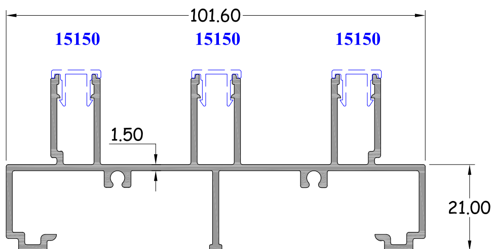
เฟรมข้าง+เฟรมบน 3 ร่อง หนา 1.5 มิล รหัสสินค้า : 15162 WT. 1.405 Kg / M.
