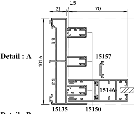
กรณีประกอบเฟรม 45 °
