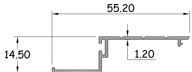
ตบธรณีขาเตี้ย รหัสสินค้า : 15107 WT. 0.227 Kg / M.
