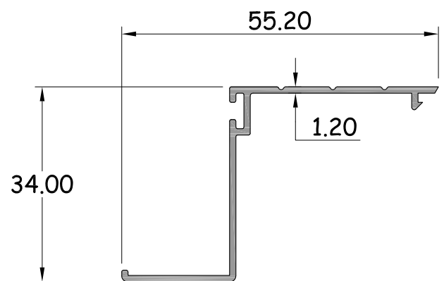
ตบธรณีขาสูง รหัสสินค้า : 15108 WT. 0.227 Kg / M.
