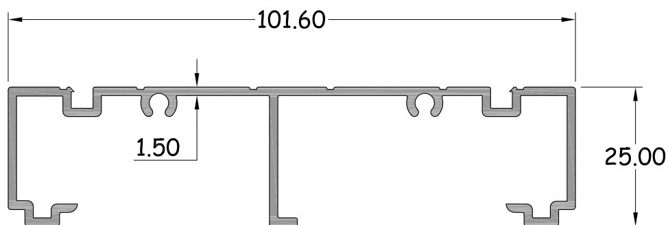
เฟรมข้าง 3 ร่อง หนา 1.5 มิล รหัสสินค้า : 15182 WT. 0.932 Kg / M.
