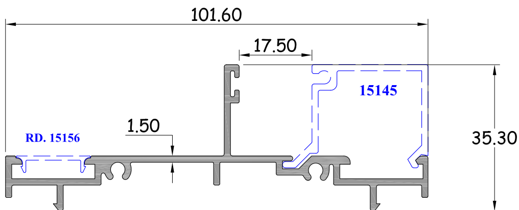
คาน C กรุ๊ป 2 ทาง หนา 1.5 มิล รหัสสินค้า : 15193 WT. 0.854 Kg / M.
