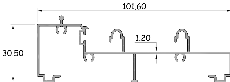
เฟรมล่างขาเตี้ย รหัสสินค้า : 15101 WT. 0.869 Kg / M.
