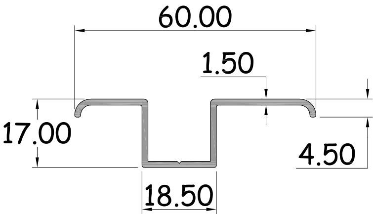
เฟรมล่างภายในบานเพ็ญ รหัสสินค้า : 15170 WT. 0.380 Kg / M.
