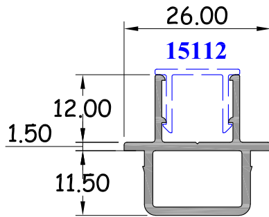
คานาบานเลื่อน หน้า 1.5 มิล รหัสสินค้า : 15163 WT. 0.343 Kg / M.
