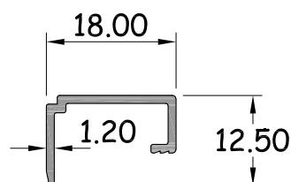
ค้ำคานาบานเลื่อน หน้า 1.5 มิล รหัสสินค้า : 15133 WT. 0.117 Kg / M.
