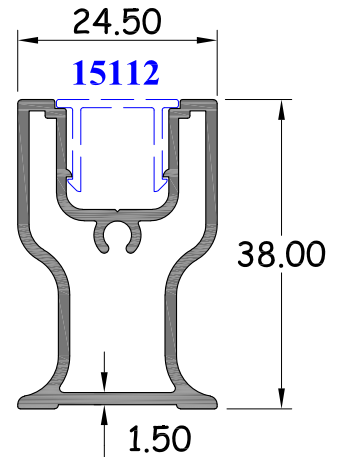
เสารับแรงบานเลื่อน (สตีฟไฟเบอร์) รหัสสินค้า : 15198 WT. 0.590 Kg / M.
