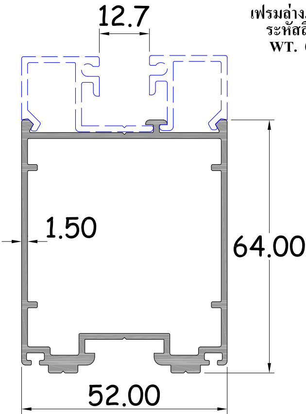
เสาบานเพ็ญ หน้า 1.5 มัด รหัสสินค้า : 15171 WT. 1.226 Kg / M.
