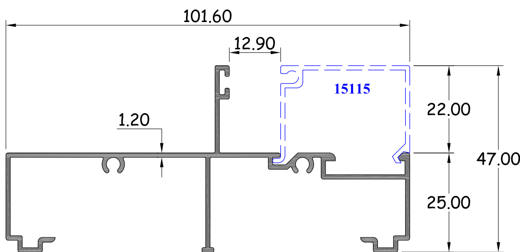
กล่องก้าน C กรูฟ รหัสสินค้า : 15200 WT. 0.795 Kg / M.
