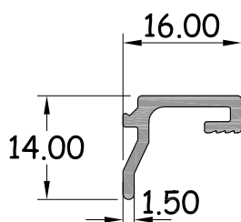
คิ้วตบกรอบบานเลื่อน หน้า 1.5 มิล รหัสสินค้า : 15148 WT. 0.148 Kg / M.
