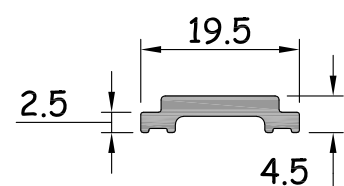
Transmission Rod รหัสสินค้า : 15157 WT. 0.145 Kg / M.
