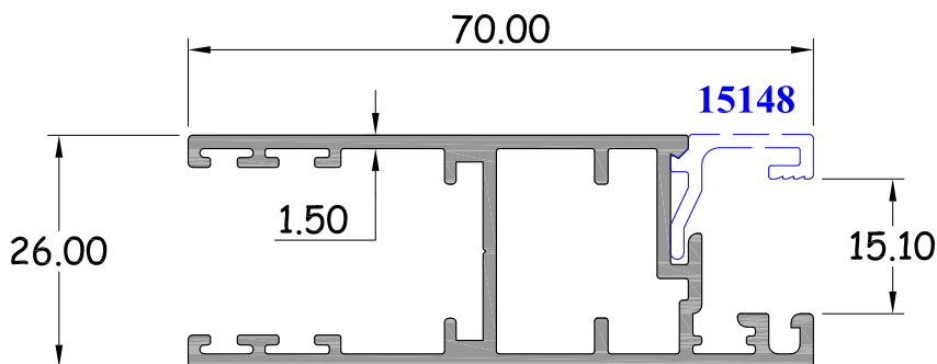
กรอบบานเลื่อนเปิดหัว 70 มิล รหัสสินค้า : 15147 WT. 0.955 Kg / M.
