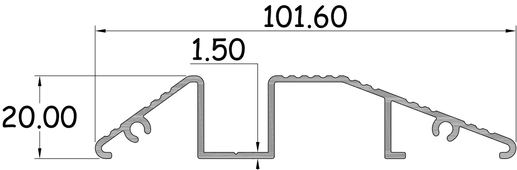
เฟรมล่างหลังเต่าบานเพ็ญ รหัสสินค้า : 15194 WT. 0.739 Kg / M.
