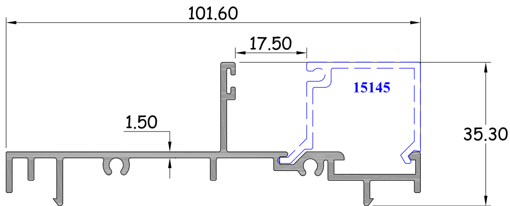
คาน C กรุ๊ป หนา 1.5 มิล รหัสสินค้า : 15160 WT. 0.848 Kg / M.
