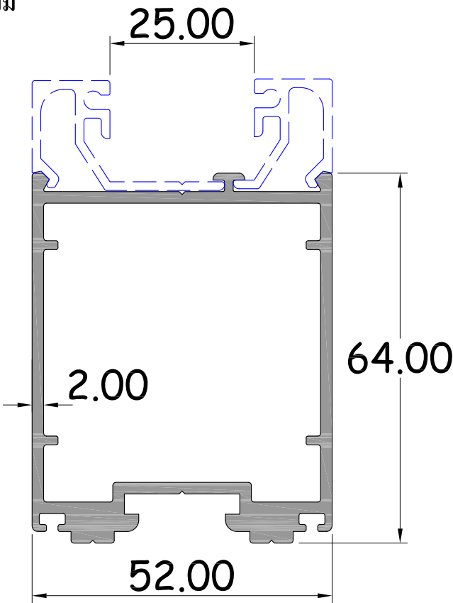
เสาบานเพ็ญ หน้า 2.0 มัด รหัสสินค้า : 15172 WT. 1.592 Kg / M.
