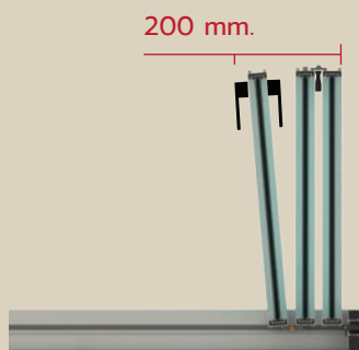
ภาพแสดงการเปิดพับสุดบาน ในฝั่งที่มีมือจับ ใช้พื้นที่ เพียง 200 mm.
