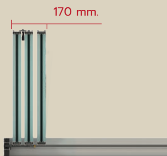
ภาพแสดงการเปิดพับสุดบาน ในฝั่งที่ไม่มีมือจับ ใช้พื้นที่ เพียง 170 mm.
