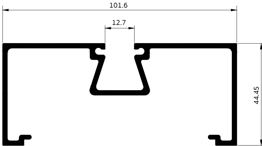
3012 กล่องร่อง 4"
