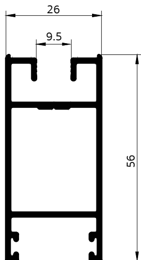
020234 เสากุญแจตัวเมีย 56 มม.
