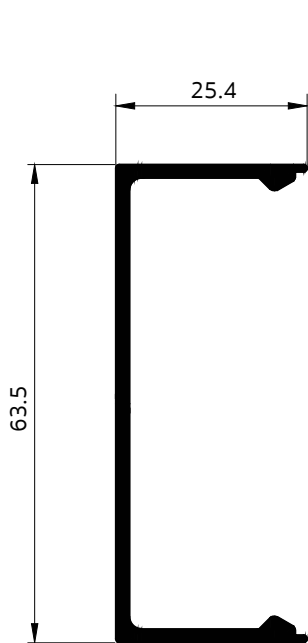
3112 ฟาเคอร์เทนวอลล์ 2"1.2 x 1
