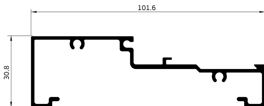
010042 กล่องเปิด (มีรูสกรู)
