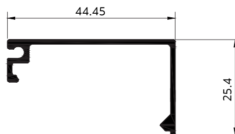
A10258 ฝาปิด-เปิด 1" (สลิม)
