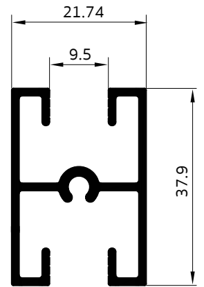
4018 เส้นแบ่งกลาง
