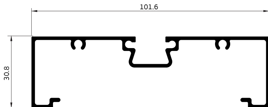
010040 กล่องร่อง (มีรูสกรู)
