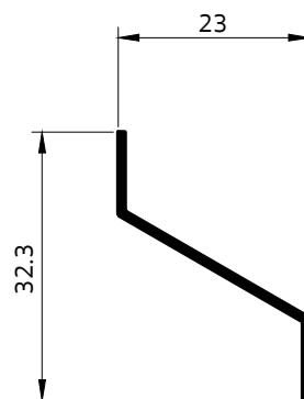
2263 แฉดเล็ก 1"
