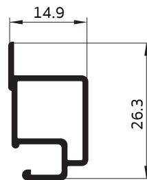
2001 เส้นหน้าต่างมีปีก
