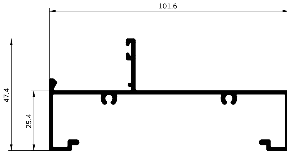
030065 กล่องก้าน 1" กระทุ้ง UN
