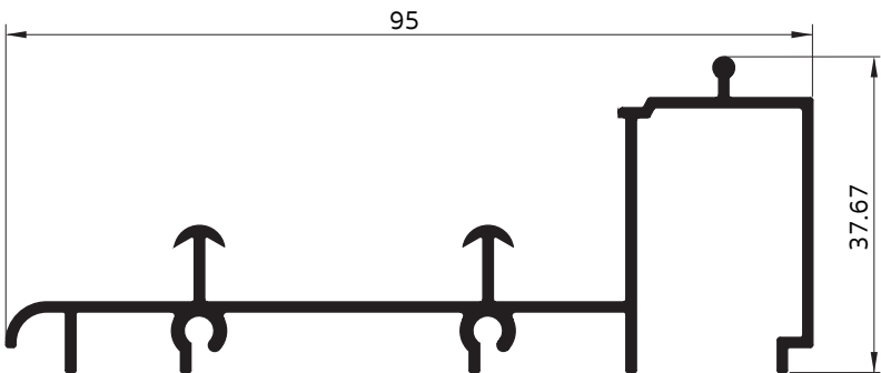
4394 เฟรมล่างขาลูง (ม
