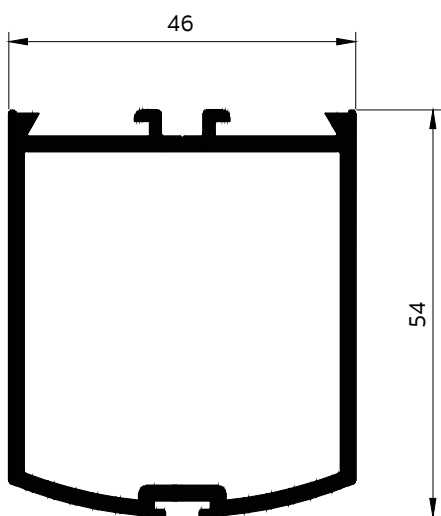
3030 เสาประตูสวิตช์
