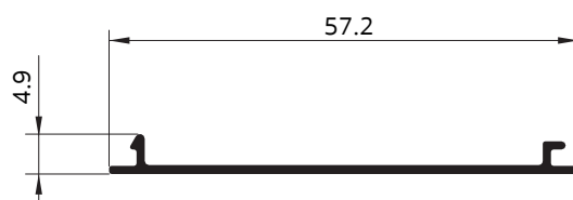
3004 ถบเรียบ 3"
