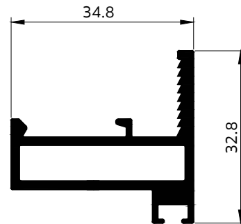
5076 กรอบนอกบานกระทุ้ง
