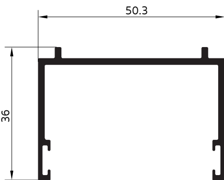
020563 เสริมเฟรมบน บิ๊กเฟรม
