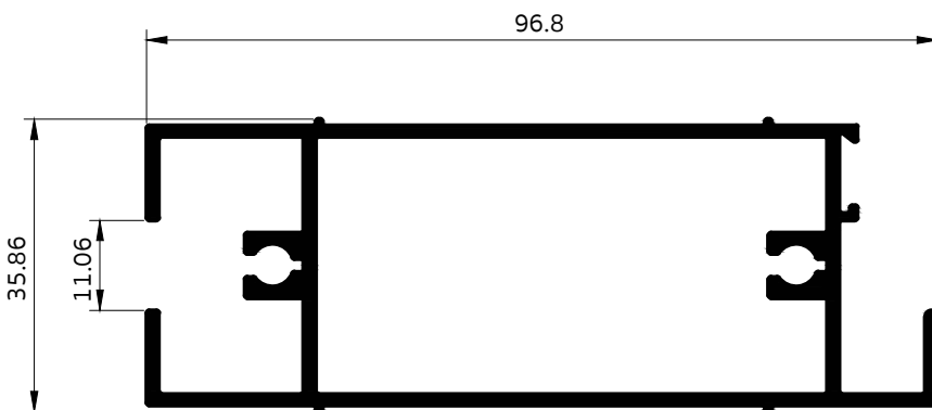
3093 เสาประตูบาน-ล่างบานเปิด 3.6"
