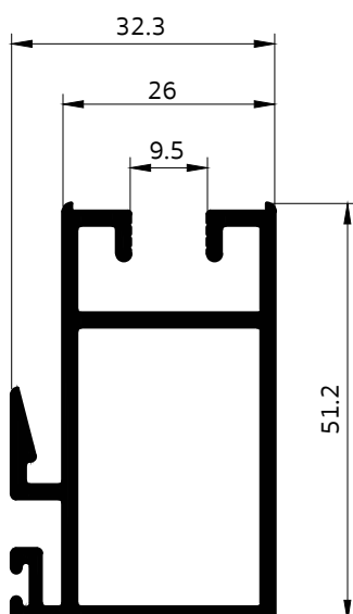
14005 เสาก๊วย 2"
