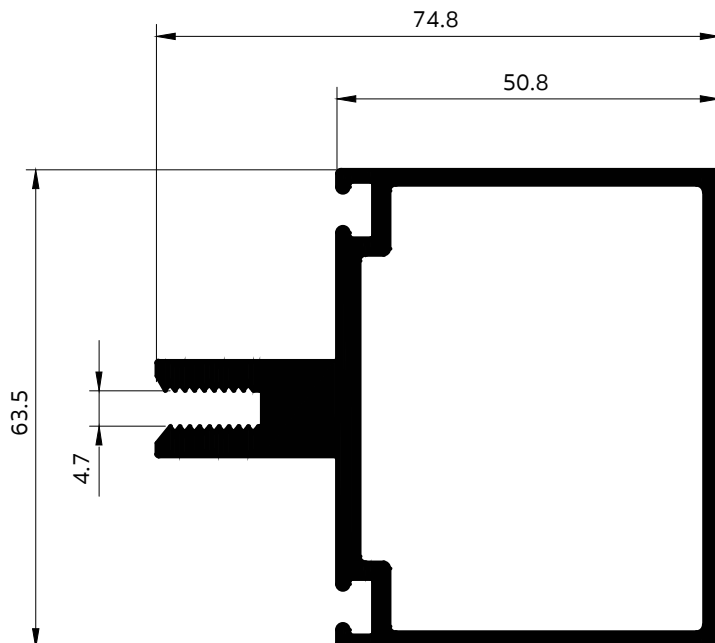
9023 เสาเคอร์เทนวอลล์ 2"1/2 x 2"
