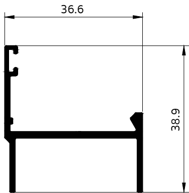
AL261 กรอบนอกหน้าต่าง UN
