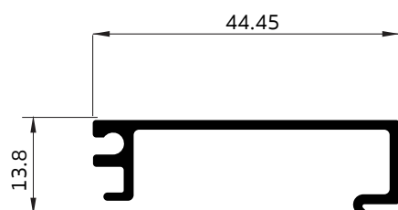
010043 ฝาเปิด-ปิด (มีรูสกรู)
