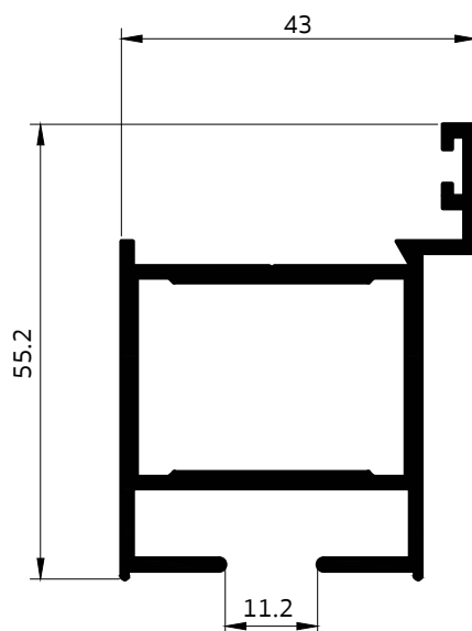
3096 เสาประตูบานเปิด 1.5" มีบังใบ
