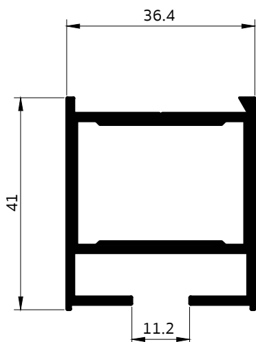
3092 เสาประตูบานเปิด 1.5"
