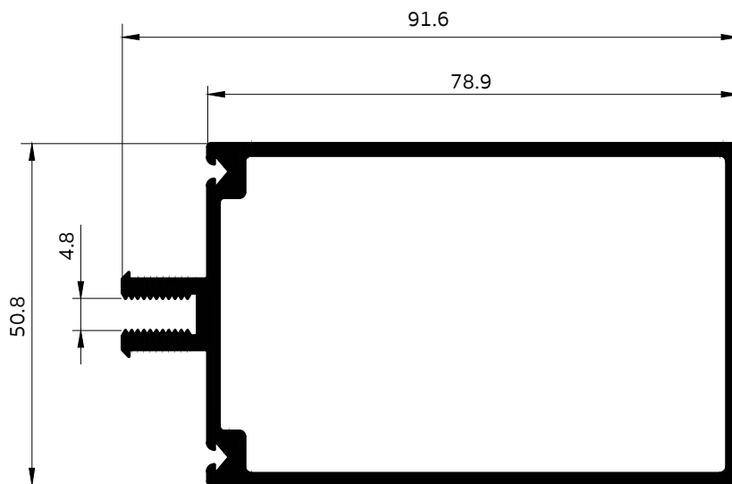
19013 เสาเคอร์วอลล์ 2" x 3"
