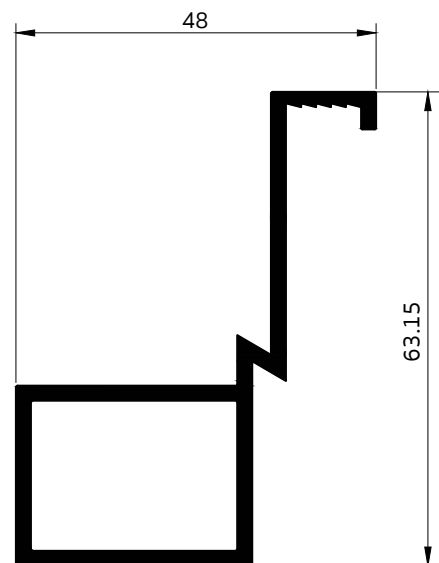
9295 กรอบบานกระทุ้ง (CURTAIN WALLS)
