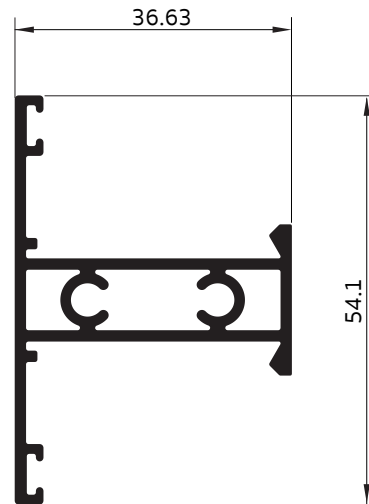
5499 ชอยกลางกระทุ้ง UN
