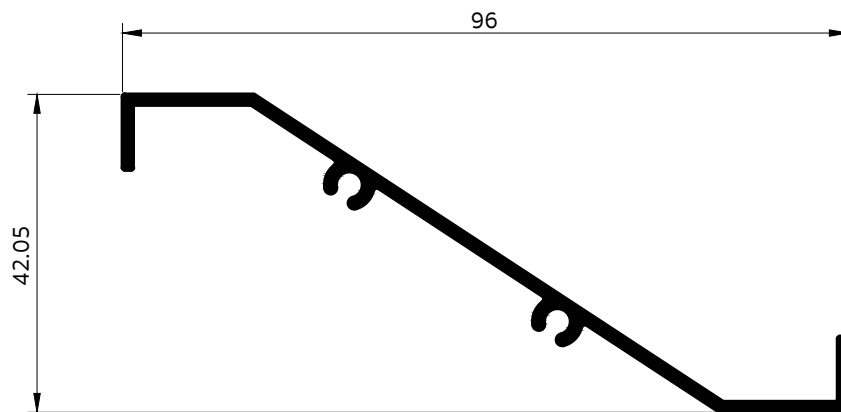
KP234 ตัว Z มีรูสกรู
