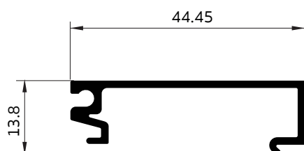
010126 ฝาปิด-ปิด 1"
