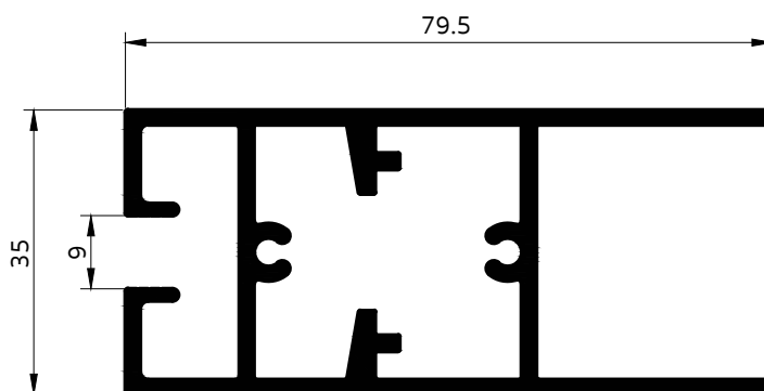
4053 ขวางล่าง นีเกอพรูม
