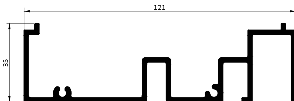
020134 รางข้างขวา
