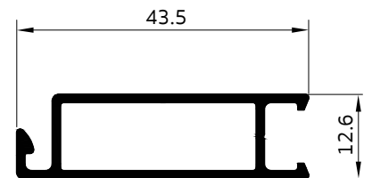
2006 กรอบมุ้ง บานเลื่อน
