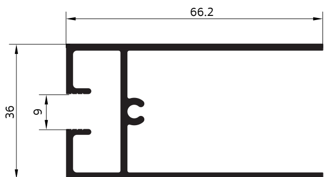
4052 ขวางล่างใน บิ๊กเฟรม
