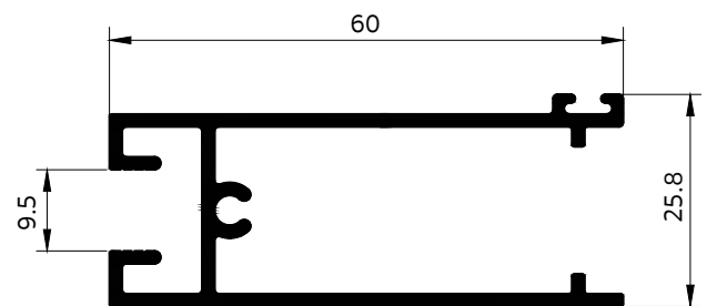
4015 ขวางล่าง บานเลื่อน
