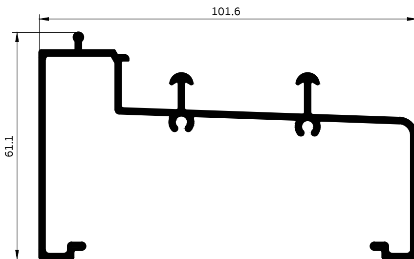
4871 เฟรมล่าง ติดกล่อง 4"
