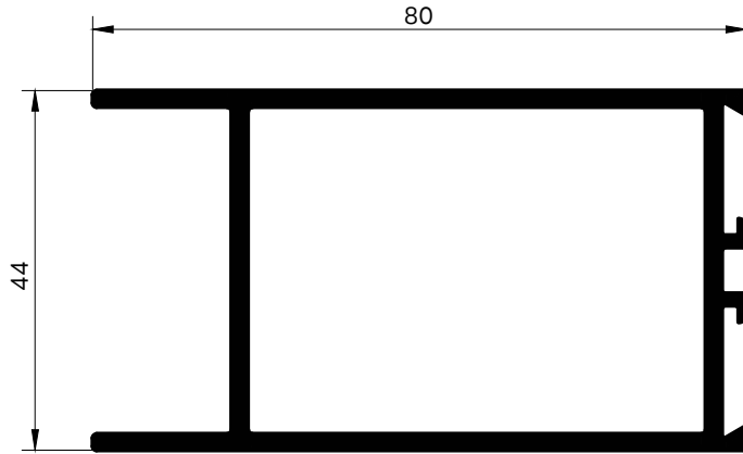
020291 ขวางบนประตูสวิง 3"
