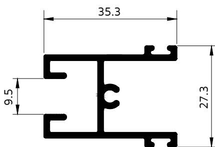
4014 ขวางบน บานเลื่อน
