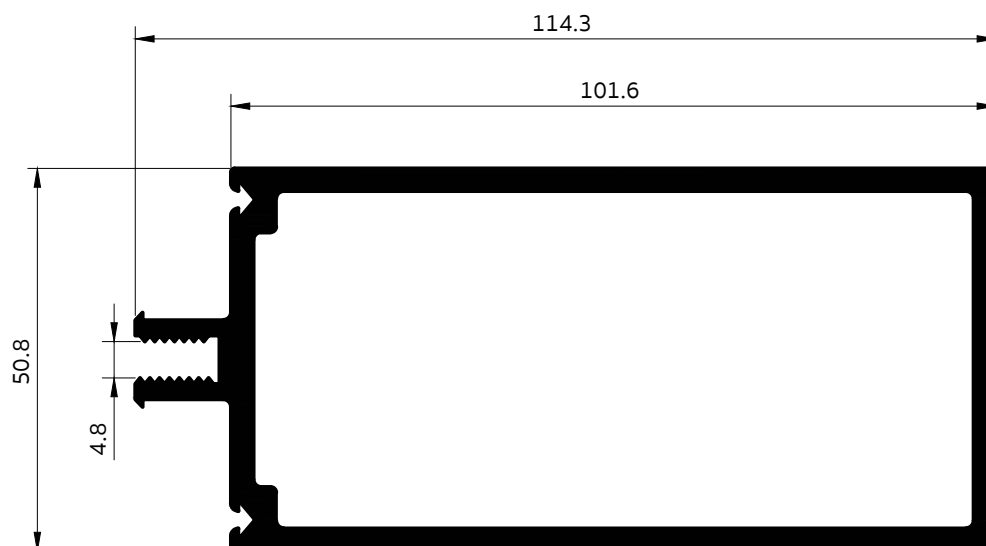
230009 เสาเคอร์วอลล์ 2" x 4"
