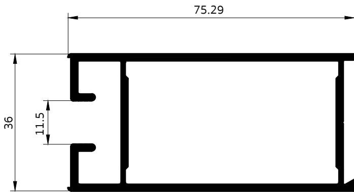
010013 เสาประตูบานพับ 3"
