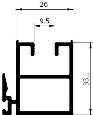
4012 เสาก๊วย
