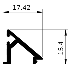
3020 คิ้วประตู
