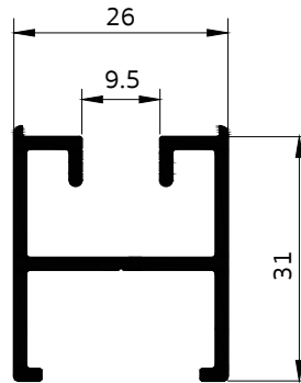
4013 เสาดาย บานเลื่อน
