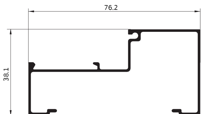
3005 กล่องเปิด 3"
