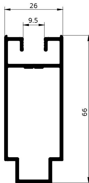
020235 เสากุญแจตัวผู้ บานเลื่อน
