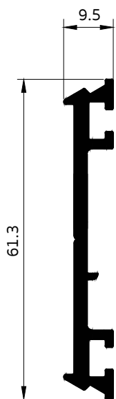
9019 ไส้เคอร์เทนวอลล์ 2.5" (ร่องยางสี่เหลี่ยม)
