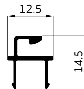
2044 เสริมมุ้งบานเลื่อน
