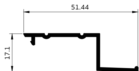
4872 ตบธรณีขาสูง (เฟรมติดกล่อง)
