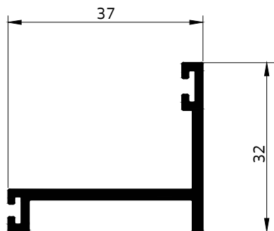
9296 กรอบนอกกระทุ้งเปลือย
