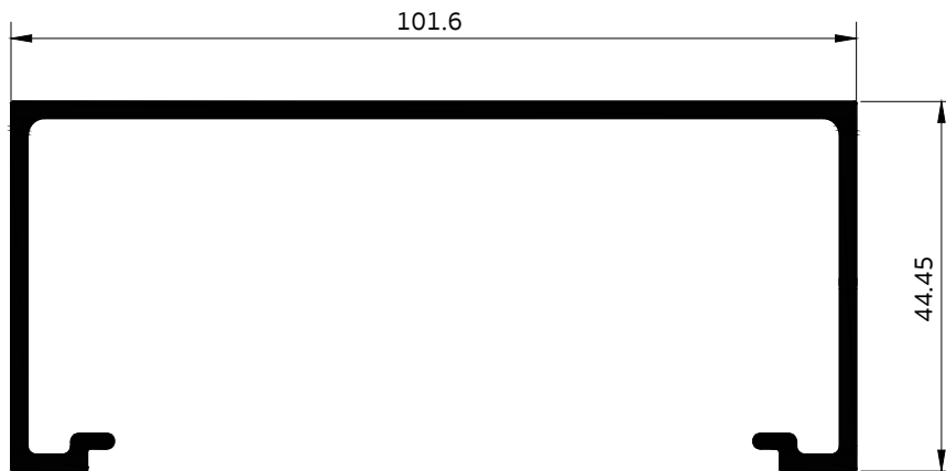
3013 กล่องเรียบ 4"
