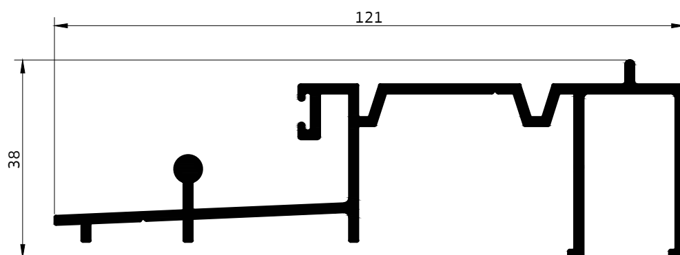
020133 เฟรมล่าง บิ๊กเฟรม มีน๊อง
