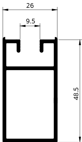
4011 เสากุญแจ บานเลื่อน
