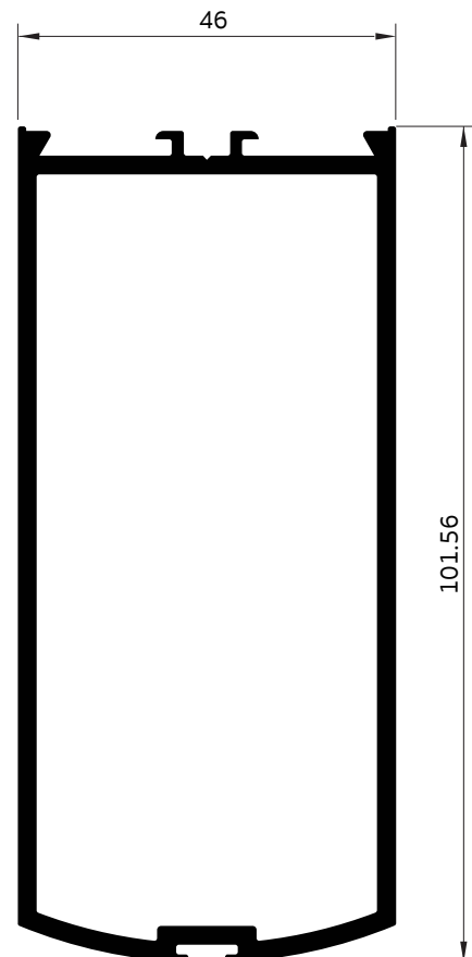
3325 เสาประตูสวิง 4"
