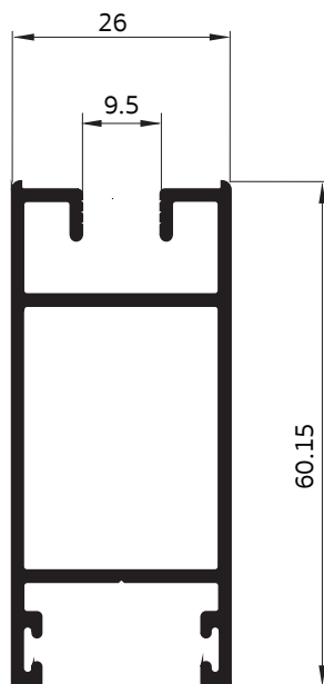
14003 เสากุญแจตัวเมีย 60 มม.
