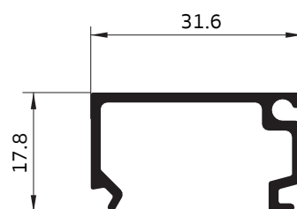
3006 ฝาเปิด-ปิด 3"
