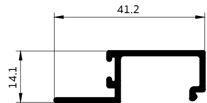
3185 คิ้วช่องแสงบานเปิด
