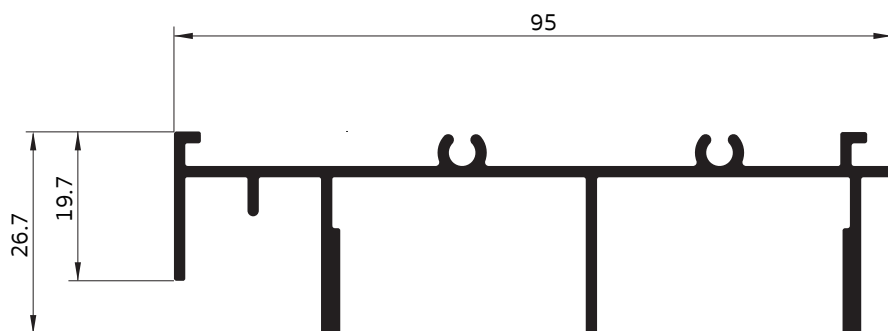
4001 เฟรมบน บานเลื่อน
