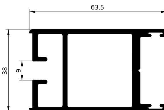
4054 เสาฤดูแฉงตัวเมีย นีเกอพรูม
