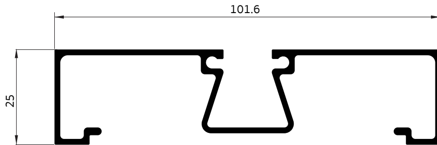
010125 กล่องร่อง 1"
