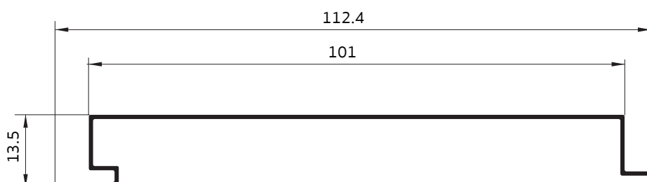
2104 ลูกฟูกเรียบชิด 4"
