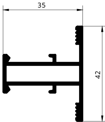
5009 ซอยกลางบานกระทุ้ง
