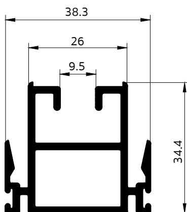
14007 เสาก๊วย 2 ทาง
