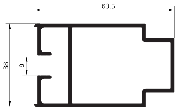
4051 เสากุญแจตัวผู้ บิ๊กเฟรม
