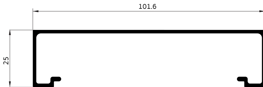
010127 กล่องเรียบ 1"
