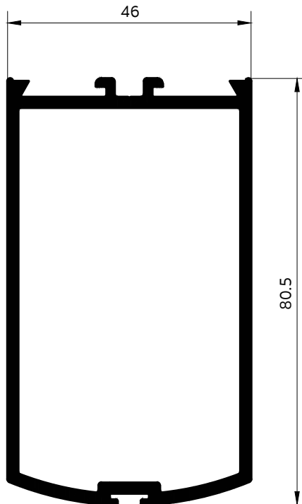
020292 เสาประตูสวิง 3"
