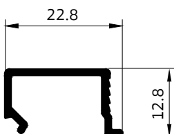
AL262 คิ้วบานกระทุ้ง UN
