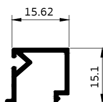
010129 คิ้วประตูเหลี่ยม
