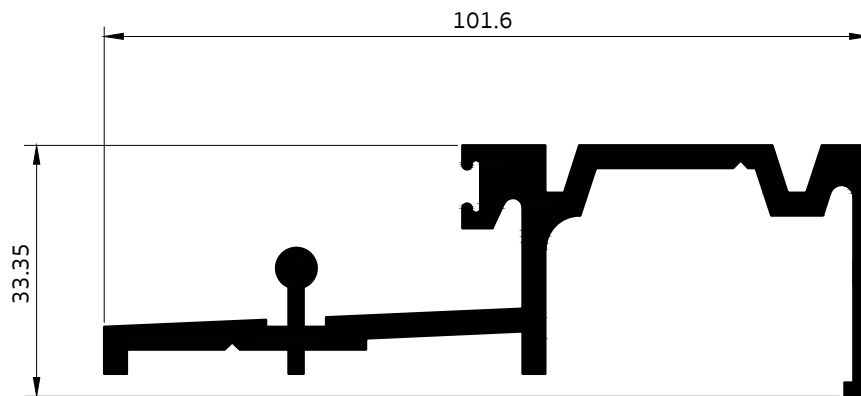
4055 เฟรมล่างบีกเฟรม
