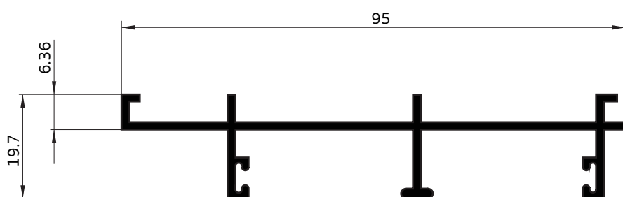
4003 เฟรมข้าง บานเลื่อน
