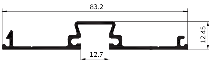
A10261 ดบร่อง 1" (สลิม)
