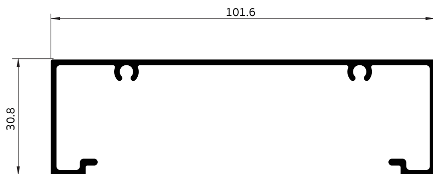
010041 กล่องเรียบ (มีรูสกรู)
