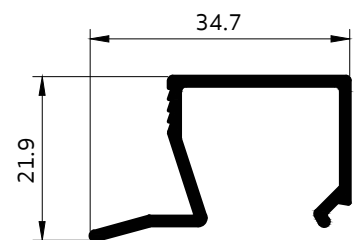
5008 คิ้วกระทุ้ง ช่องแสง UN
