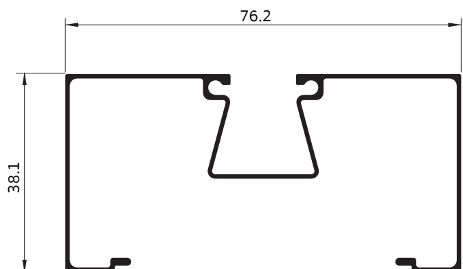
3001 กล่องร่อง 3"
