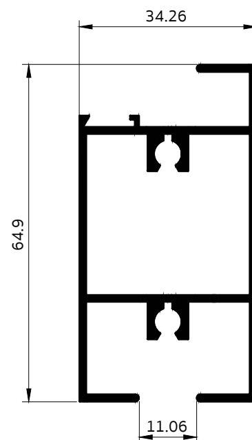
3094 เสาประตูบาน-ล่าง บานเปิด 2.5"
