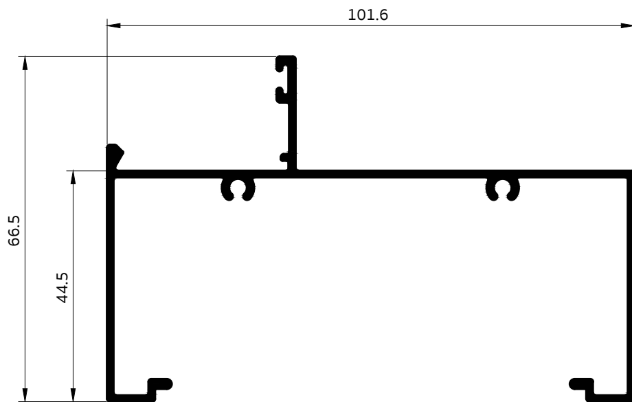
030131 กล่องก้าน 1" 3/4 กระทุ้ง UN
