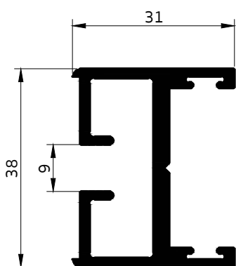
4057 เสาดาย นีเกอพรูม
