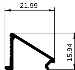
5005 คิ้วบานกระทุ้ง
