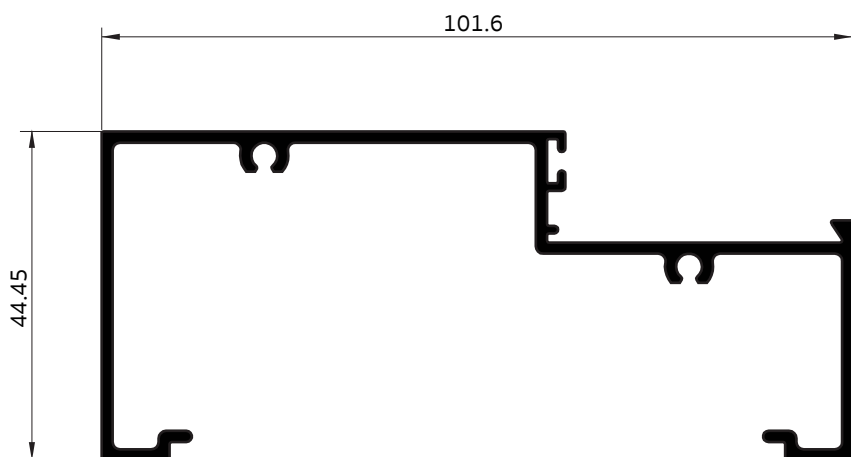
010076 วงกบไม้ (มีรูสกรู)
