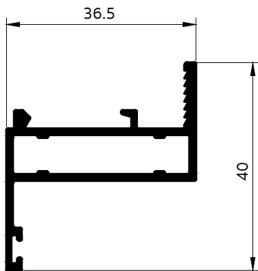
5025 กรอบนอก กระทุ้ง UN
