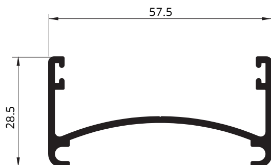
3344 ชนกลางรางแขวน
