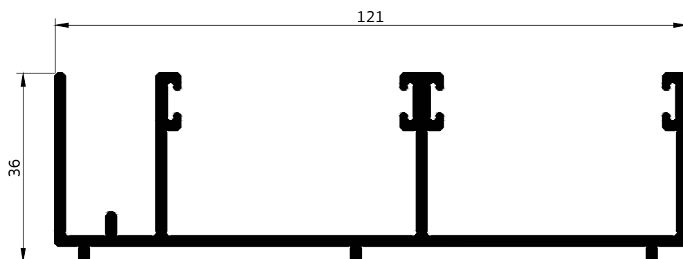
020132 เฟรมบน บิ๊กเฟรม มีน๊อง
