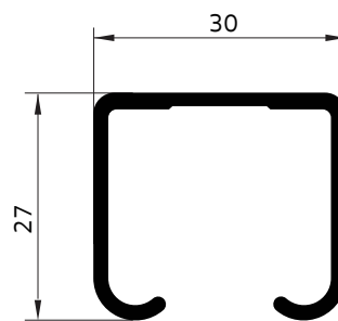
3061 รางแขวนเล็ก
