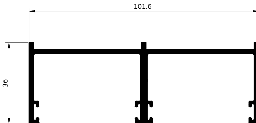
4056 เฟรมบนบีกเฟรม
