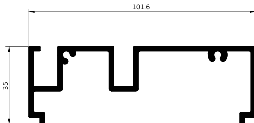
4058 เฟรมข้างบีกเฟรม
