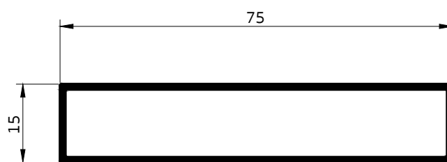
110011 รู Grill 75x15 mm
