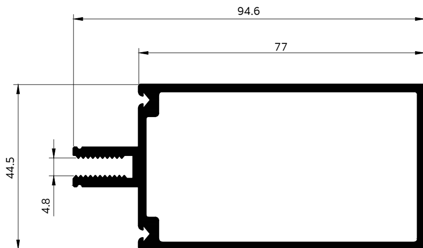
9013 เสาคอร์เทนวอลล์ 1"3/4 x 3"
