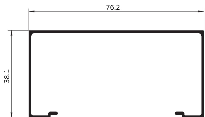
3002 กล่องเรียบ 3"
