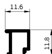
3095 คิ้วประตูบานเปิด
