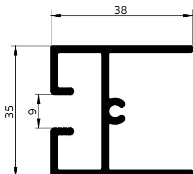
4060 ขวางบน นีเกอพรูม
