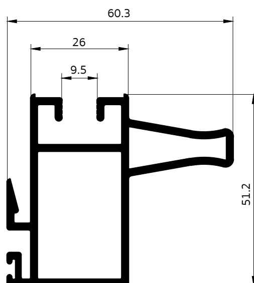
14091 เสาก๊วยมือจับ 2"
