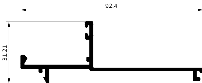
030064 ฟาตบกล่องก้าน กระทุ้ง UN
