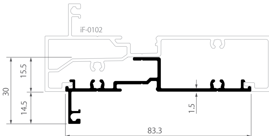
iF-0104 ตาช่องแสง ไอคอนิก 0.661 kg/m
