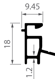
iS-0205 เสริมมุมบานเลื่อน ไอคอนิก 0.180 kg/m
