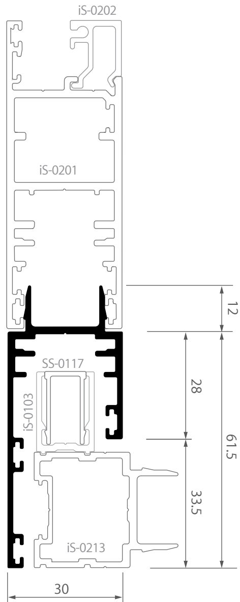
iS-0212 อะแดปเตอร์ต่อมุม บานลิ้น ไอคอนิก 0.805 kg/m
