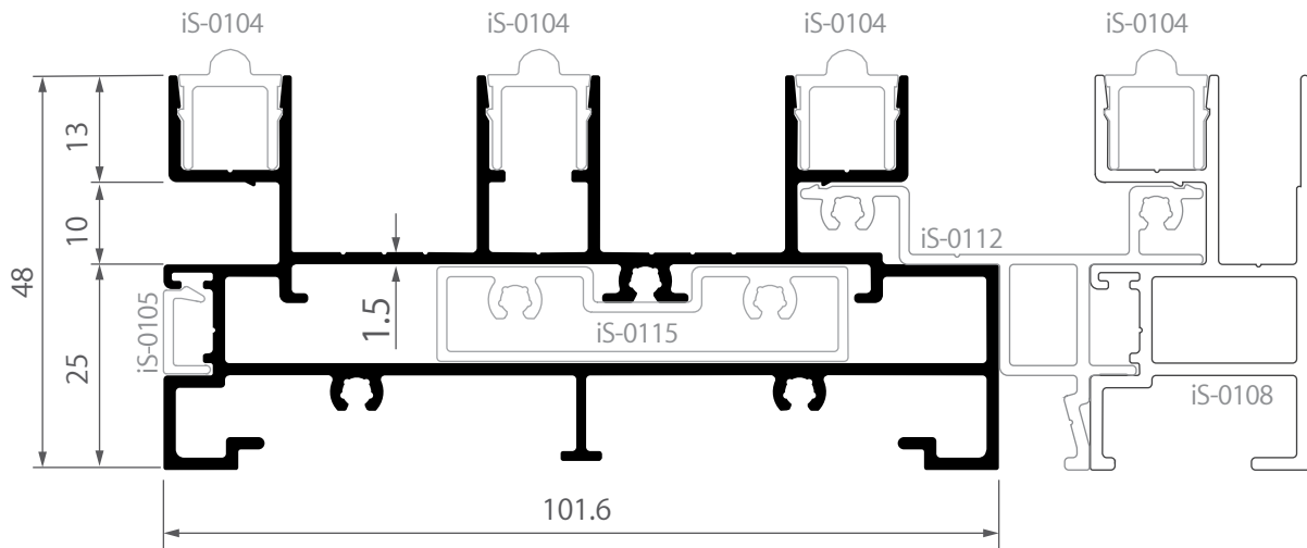
iS-0101 เฟรมบน-ล่างบานเลื่อน ไอคोनิก 1.899 kg/m
