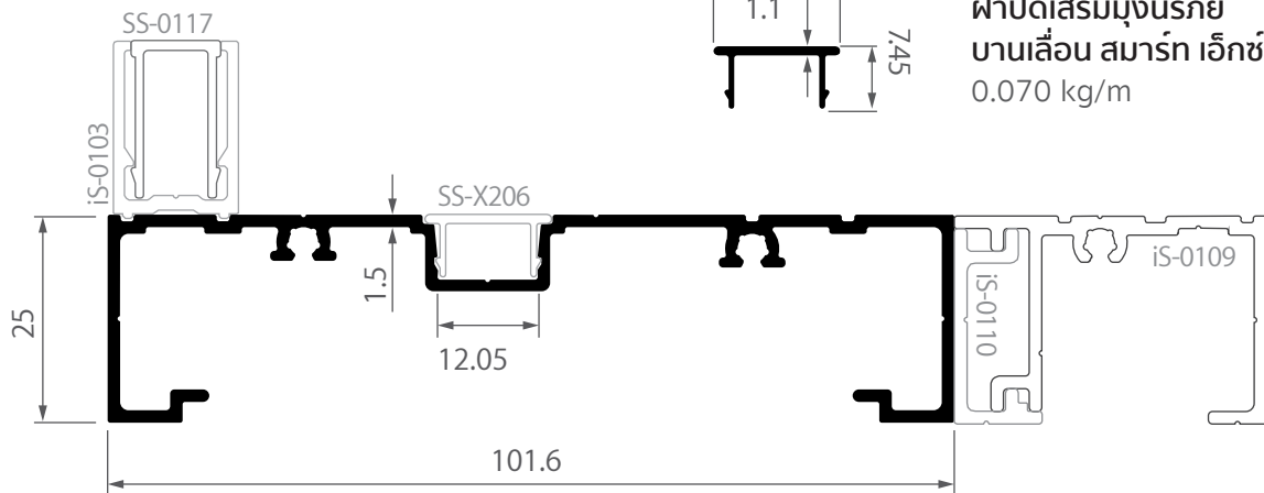
iS-0102 เฟรมข้างบานเลื่อน ไอคोनิก 0.869 kg/m
