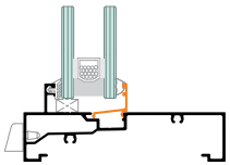
คิ้วร่องกระจก 33.5 มม. ใส่กระจก 26 - 30 มม.
