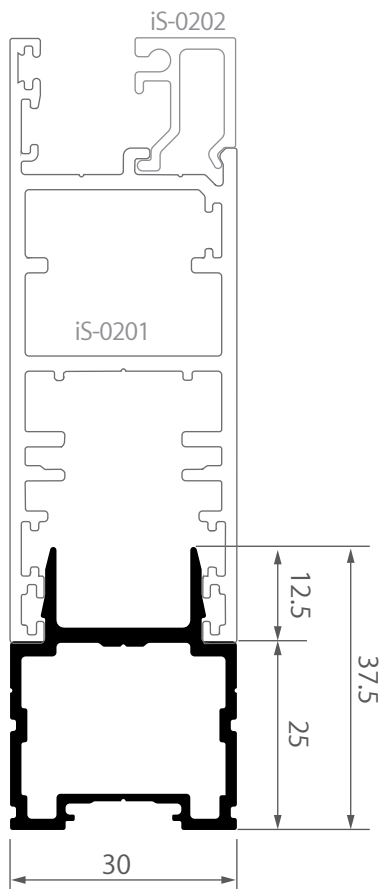
iS-0213 อะแดปเตอร์ต่อมุม บานรอง ไอคอนิก 0.600 kg/m
