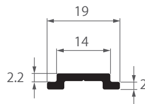
030038 ก้านสไลด์ บัลตีพอยท์ล็อก 0.126 kg/m
