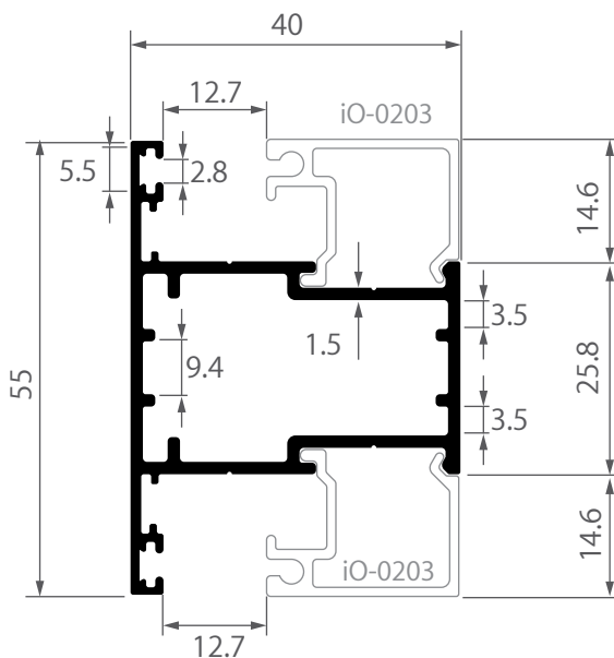
iC-0202 ซอกรอบบานกระทุ้ง ไอคอนิก 0.765 kg/m
