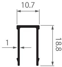
SS-0117 ฝาปิดเสริมเสา กฤษณาตัวผู้ สมาร์ท 0.135 kg/m
