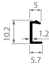
iS-0105 ฝาปิดระบายน้ำ หน้าเฟรม ไอคอนิก 0.057 kg/m
