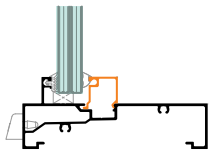
คิ้วร่องกระจก 20 มม. ใส่กระจก 10 - 16 มม.
