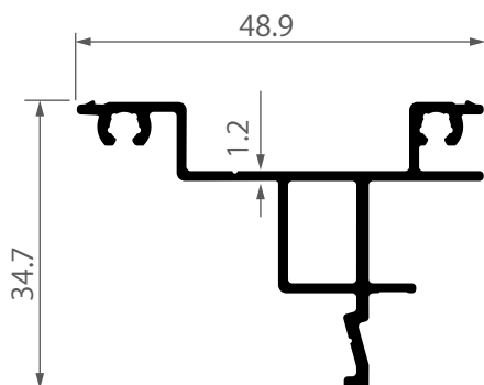
iS-0112 ตัวต่อเฟรมฝังใน บานเลื่อน ไอคอนิก 0.496 kg/m
