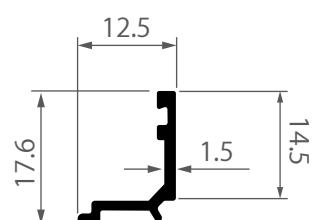
iS-0204 คิ้วกรอบบาน 2.0 ร่องกระจาก 23.5 มม. ไอคอนิก 0.122 kg/m
