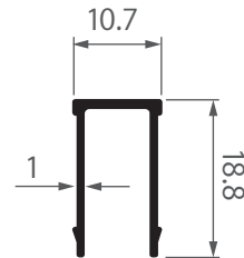
SS-0117 ฝาปิดเสริมเสา ทุจั่วตัวผู้ สมาร์ท 0.135 kg/m
