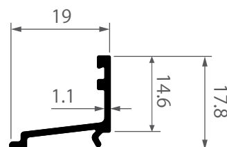
iO-0205 คิวกรอบบาน 33.5 ไอคอนิก 0.134 kg/m
