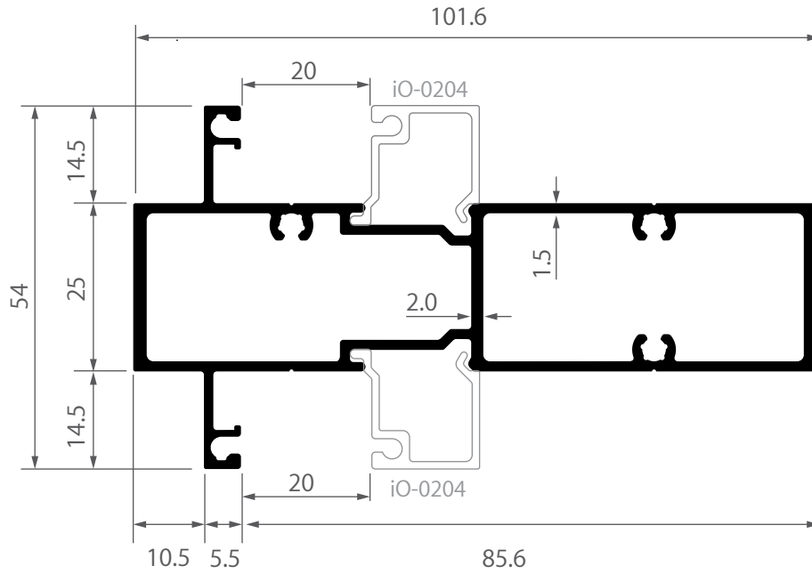
iF-0103 ชอยเฟรมช่องแสง ไอคอนิก 1.513 kg/m
