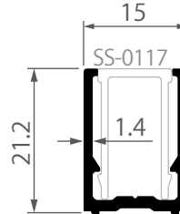
iS-0103 ยูเสริมปีกเฟรมข้าง บานเลื่อน ไอคอนิก 0.230 kg/m
