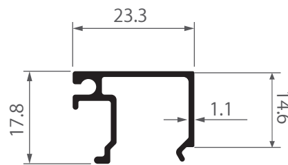
iO-0203 คิวกรอบบาน 12.7 ไอคอนิก 0.222 kg/m
