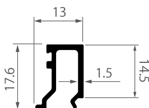
iS-0203 คิ้วกรอบบาน 2.0 ร่องกระจาก 16 มม. ไอคอนิก 0.179 kg/m
