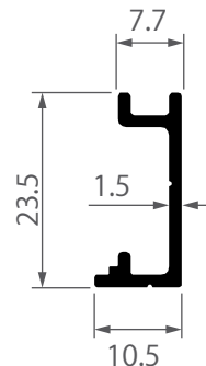
iS-0110 ปิดเฟรมข้างบานเลื่อน รางเดี่ยว ไอคอนิก 0.182 kg/m
