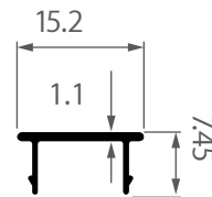
SS-X206 ฝาปิดเสริมมุ้งนิรภัย บานเลื่อน สมาร์ท เอ็กซ์ 0.070 kg/m
