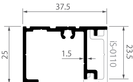
iS-0109 เฟรมข้างบานเลื่อน รางเดี่ยว ไอคอนิก 0.450 kg/m
