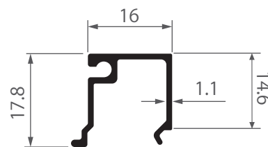
iO-0204 คิวกรอบบาน 20 ไอคอนิก 0.186 kg/m
