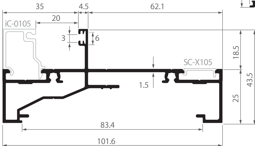
SC-X106 เสริมช่องแสงเฟรมบานกระทุ้ง สมาร์ท เอ็กซ์ 0.426 kg/m
