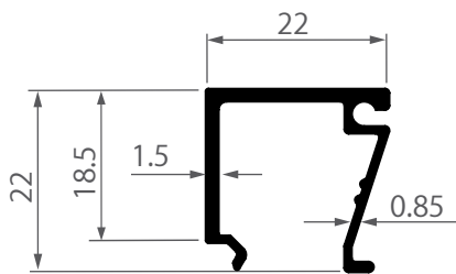
A30274 คิวช่องแสง เฟรมกระทุง 12.7 พรีเมียม 0.250 kg/m
