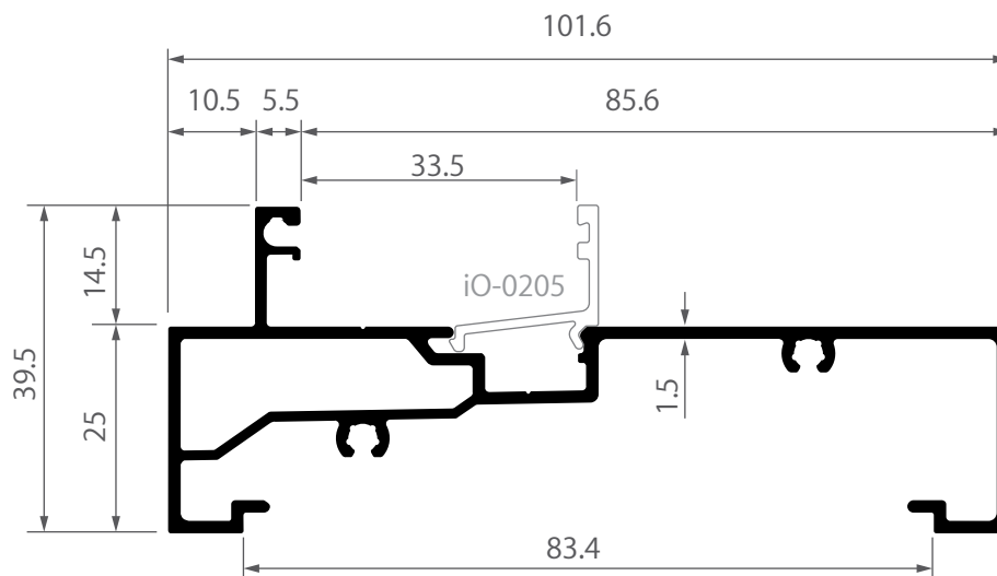
iF-0102 เฟรมล่างช่องแสง ไอคอนิก 1.077 kg/m
