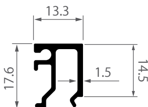
iS-0202 คิ้วกรอบบาน 2.0 ร่องกระจาก 12.7 มม. ไอคอนิก 0.211 kg/m
