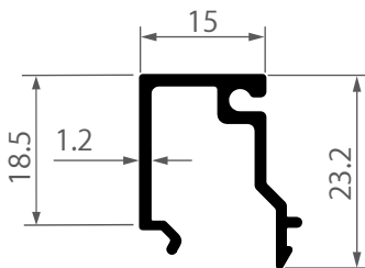
iC-0105 คิวช่องแสง เฟรมกระทุง 20 ไอคอนิก 0.218 kg/m
