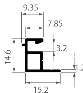
SC-X202 เสริมบุ้งบานกระทุ้ง สมาร์ท เอ็กซ์ 0.160 kg/m
