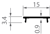
iS-0209 ฝาปิดสกรูตบเกี่ยว ไอคอนิก 0.047 kg/m
