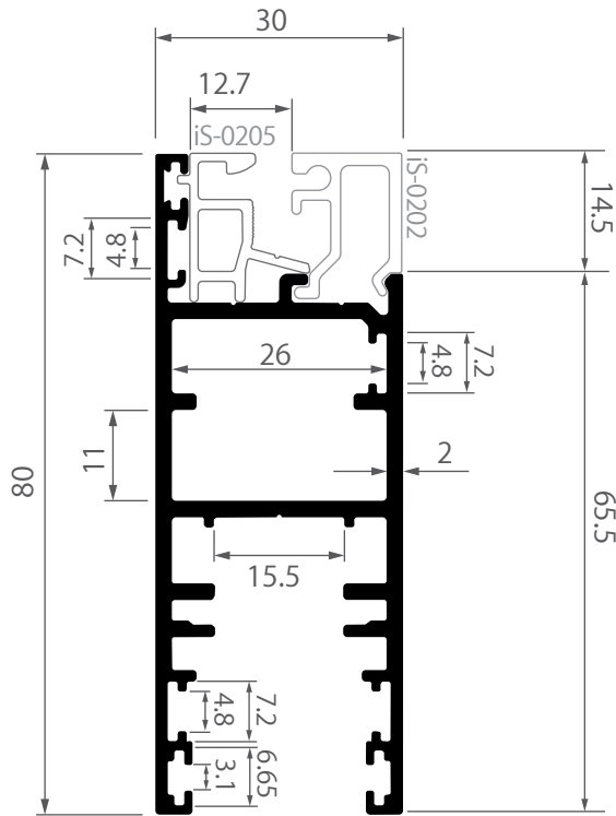
iS-0201 กรอบบานเลื่อน 2.0 ไอคอนิก 1.322 kg/m
