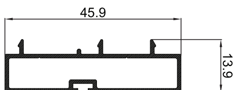
P-003588 ฝาครอบกรอบบาน ด้านล่าง
