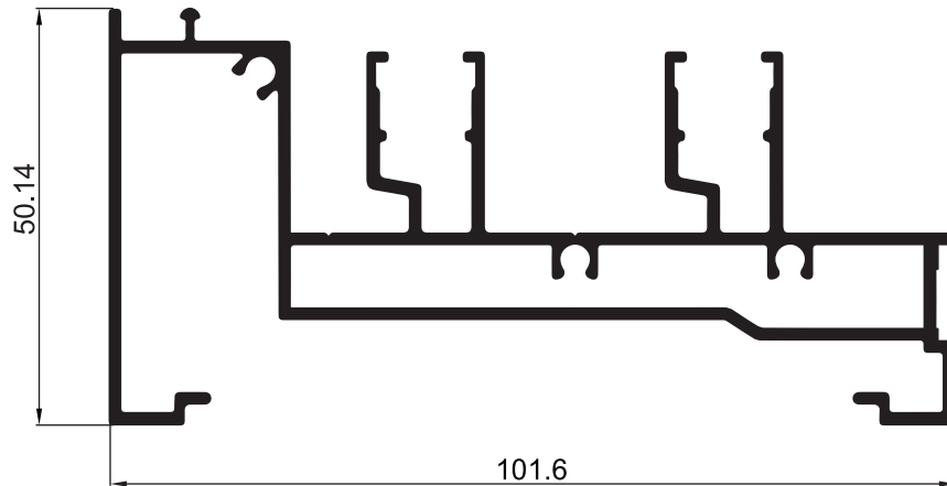
NEW P-124563 / 154465 เฟรมบน-ล่างบานเลื่อน 4" ( 2 ราง )
