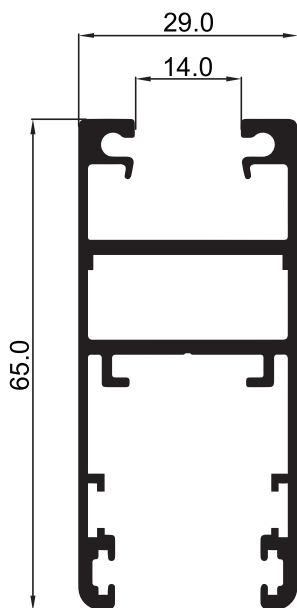
P-134573 กรอบบานมัลติล็อค ER ร่องลึกหลายด 5x5 มม.
