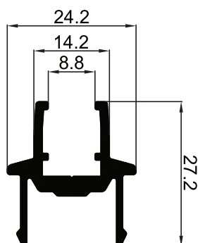
P-009414 ชนกลางบานเลื่อน
