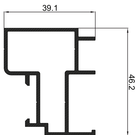
P-003770 ชนกลางประตูบานเปิดคู่ ER
