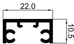
P-003763 เสริมรางเฟรมล่างยุโรป
