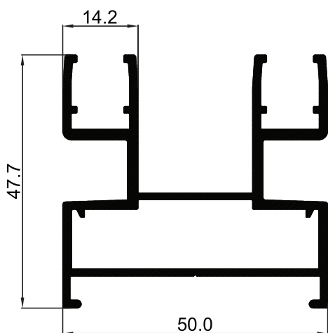
P-124561 / 009519 เฟรมบานเลื่อน 2 ราง
