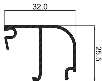
P-009518 คิ้ว 50c
