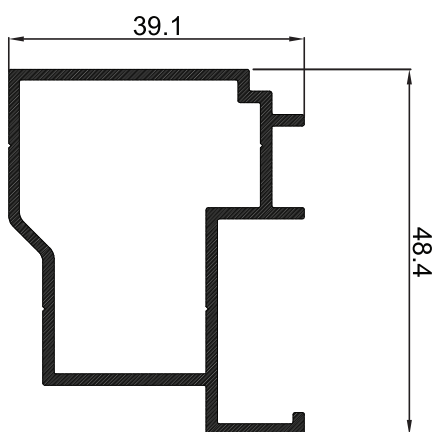
P-003233 กรอบบานเปิด ER 4"
