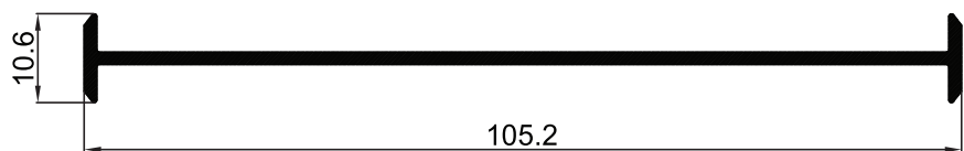
P-003589 ตัวต่อวงกบเล็ก 4"
