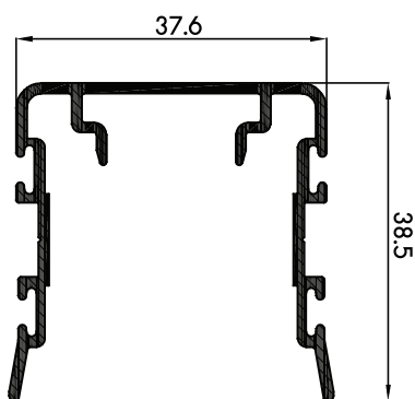
P-133106 ตบเกี่ยว 2 ทาง ร่องลึกหลาดคู่
