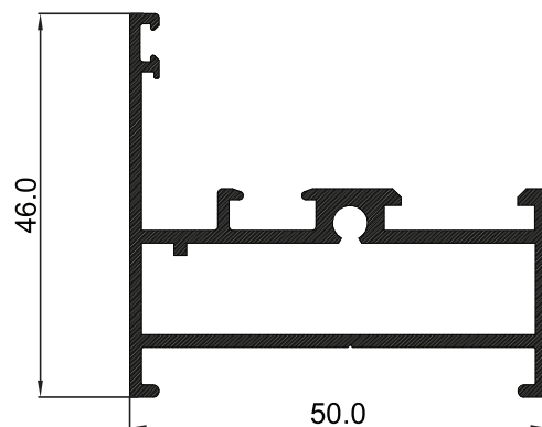
P-003603 เฟรมล่างประตูบานเปิด
