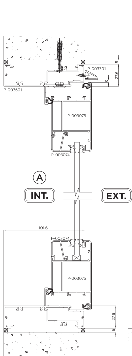
เฟรมบาน-ล่าง หน้าต่าง ขนาด 4"
