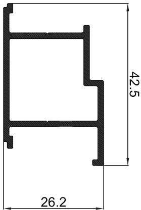
P-003591 ชนกลางบานเปิด
