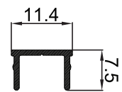
P-003696 ฝ้าตบเฟรมล่างประตู บานเปิด ER
