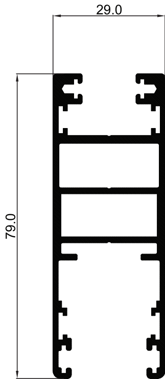
P-003766 กรอบบานยูโร Multi
