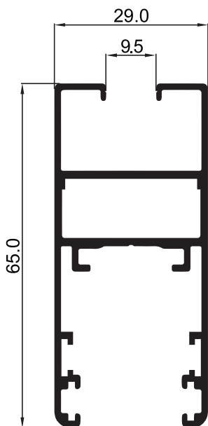
NEW P-154558 กรอบบาน
