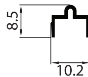
NEW P-104311 รางล้อภายใน
