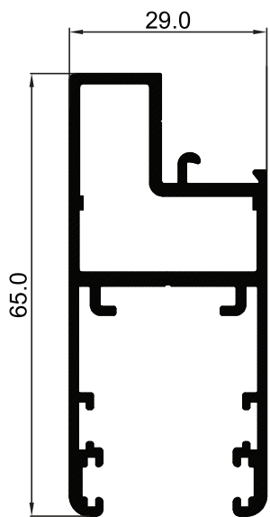
P-003590 กรอบบาน
