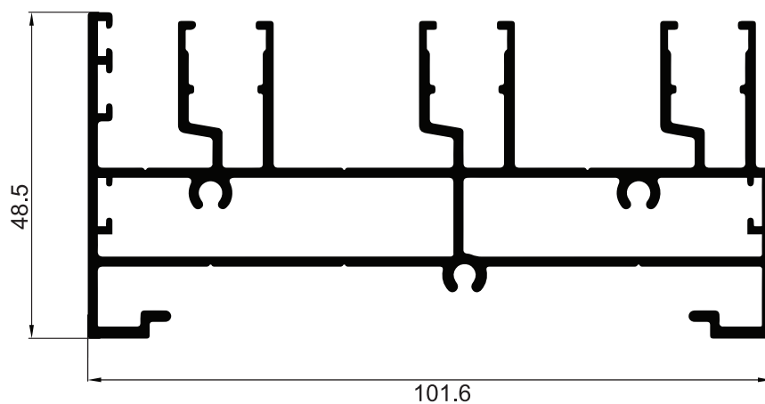
NEW P-124562 / 154307 เฟรมบานเลื่อน 4" ( 3 ราง )
