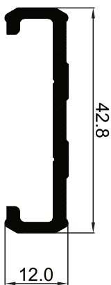
P-009413 ไส้ต่อบาน fix
