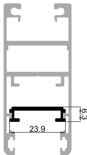
P-007227 ซีเสริมบาน ER
