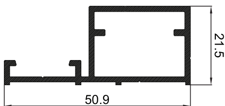
P-003595 ตัวต่อเฟรมบานเปิด
