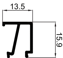
P-003592 คิ้ว
