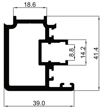
P-003764 เสาเข้ามุมยูโร Multi
