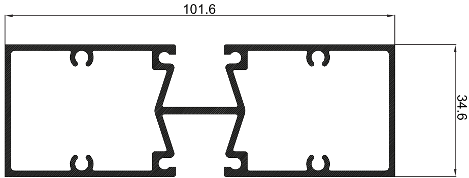
P-003092 กล่องร่องสองด้าน ER
