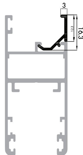
P-123119 คิ้ว (ระยะ 20 มม.)
