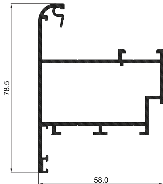
P-009517 กรอบบานหน้าต่าง ER 50c
