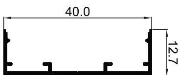
P-003142 ยูแคป Capping เล็ก
