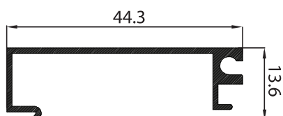
P-158432 กล่องเปิด
