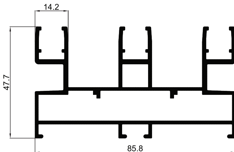
P-009509 เฟรมบานเลื่อน 3 ราง
