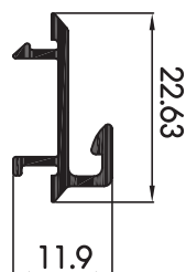
P-003592 คิ้ว
