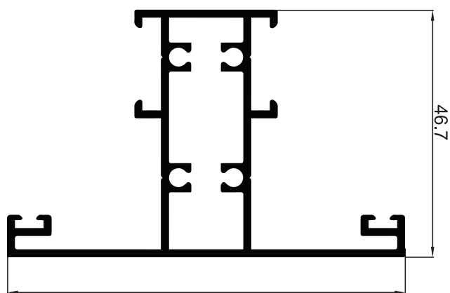
NEW P-154516 แบ่งกระจก
