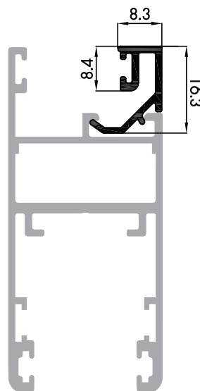
P-123118 คิ้ว (ระยะ 10 มม.)
