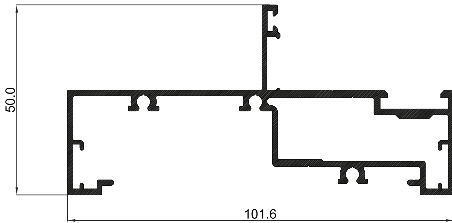
P-003601 เฟรมบานเปิด
