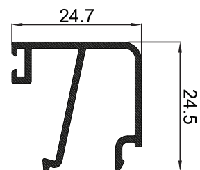
P-003074 คิ้วบานเปิด ER 4"
