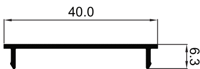
P-003400 ฝาแคป Capping
