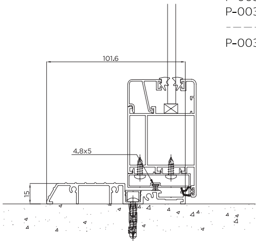
เฟรมล่างประตู ขนาด 4"
