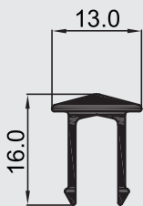
P-009511 รางล้อ บน-ล่าง
