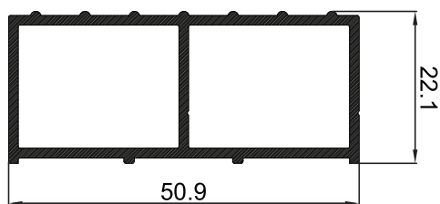
P-003593 ตัวต่อเฟรมล่างบานเปิด
