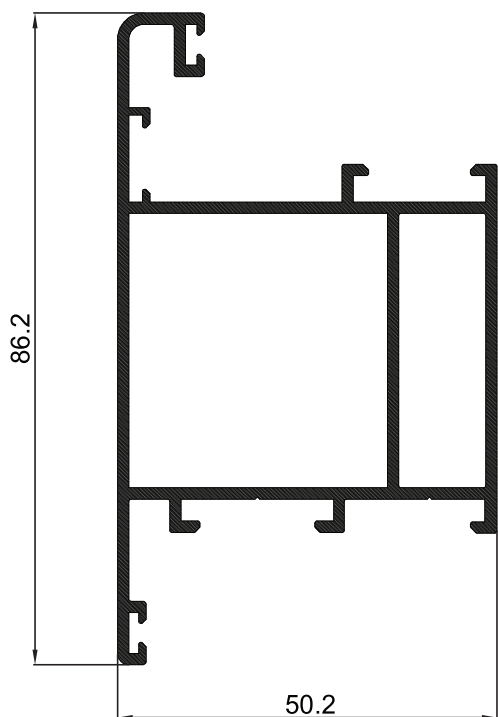
P-003075 กรอบบานเปิด ER 4"
