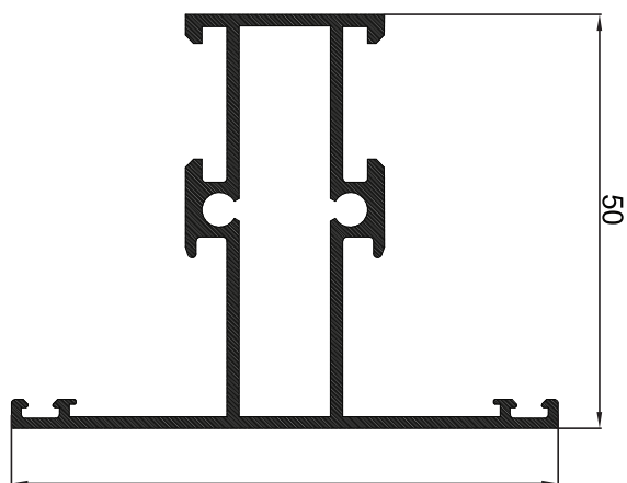
P-007225 แบ่งบาน ER 50c
