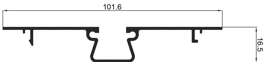
P-003093 ถบร่องขยายว ER
