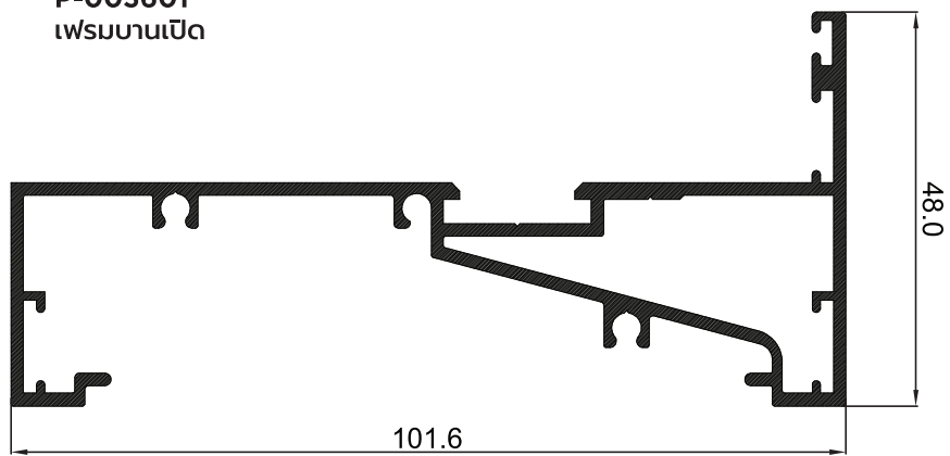
P-006964 เฟรมวงกบคิ้วใน ER 4"
