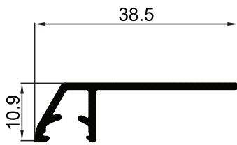
P-003594 Headsill ขายาว
