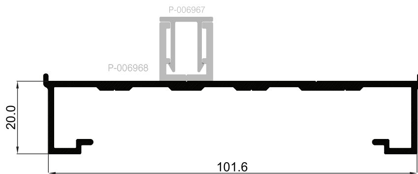
P-124560 / 006969 เฟรมข้างบานเลื่อน 4"
