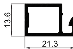
P-003596 กรอบบานมุ้ง
