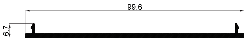
P-003587 ตัวต่อวงกบใหญ่ 4"
