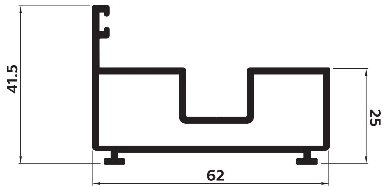
P-157935 เฟรมวงกบ ล่าง (ภายนอก)
