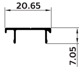
NEW P-104142 ฝาพับเฟรมข้าง
