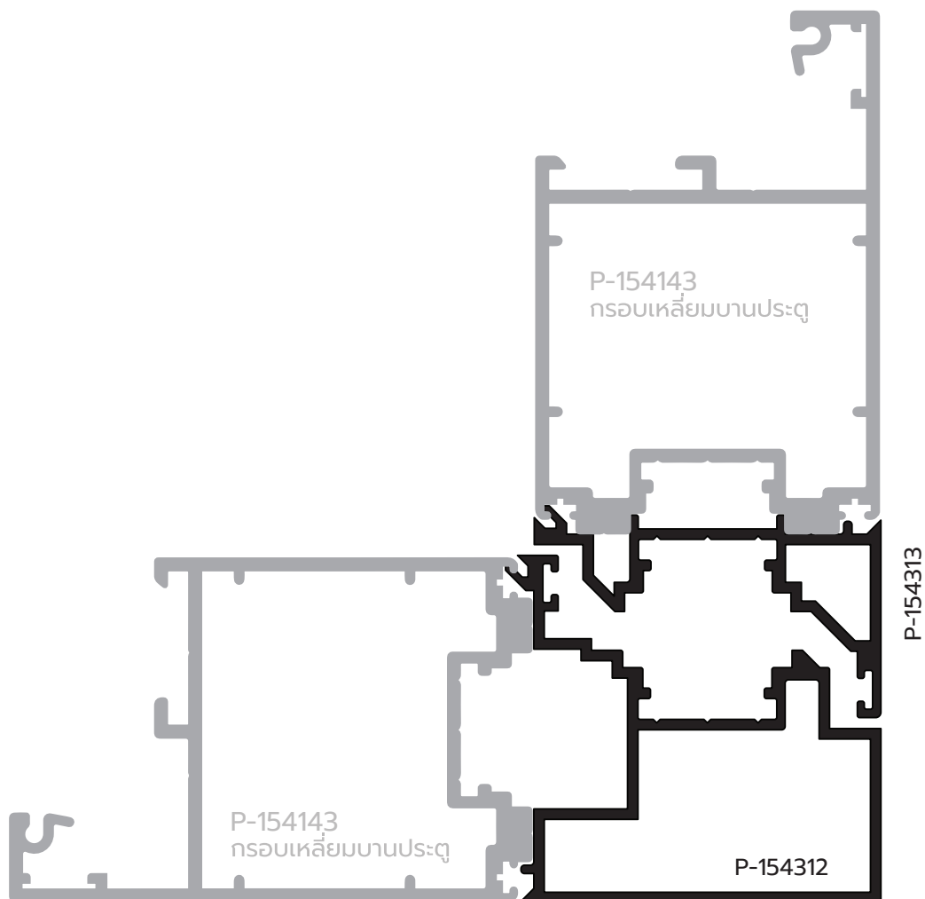
NEW P-154312 เสาเข้ามุม
