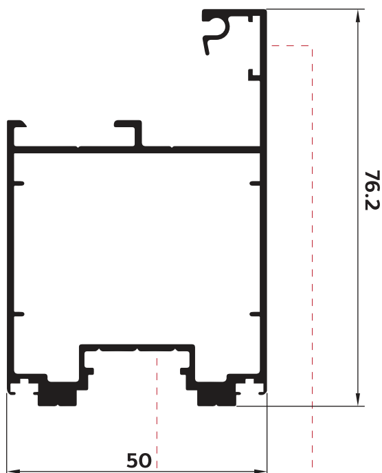
NEW P-154143 กรอบเหล็บบานประตู
