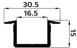
NEW P-204147 รางยูแบบฝัง
