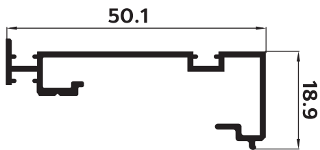
P-107294 ฝาตบกลางบานเพิ่ม หัวเหลี่ยม
