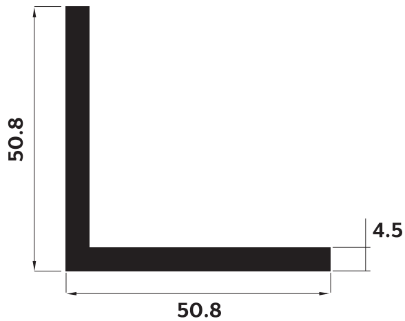
P-457434 จากข้อต่อ 2x2"
