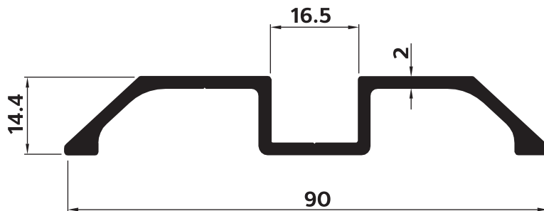
P-208901 เฟรมวงกบ ล่าง (ภายใน)
