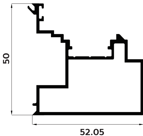
NEW P-154312 เสาเข้ามุม
