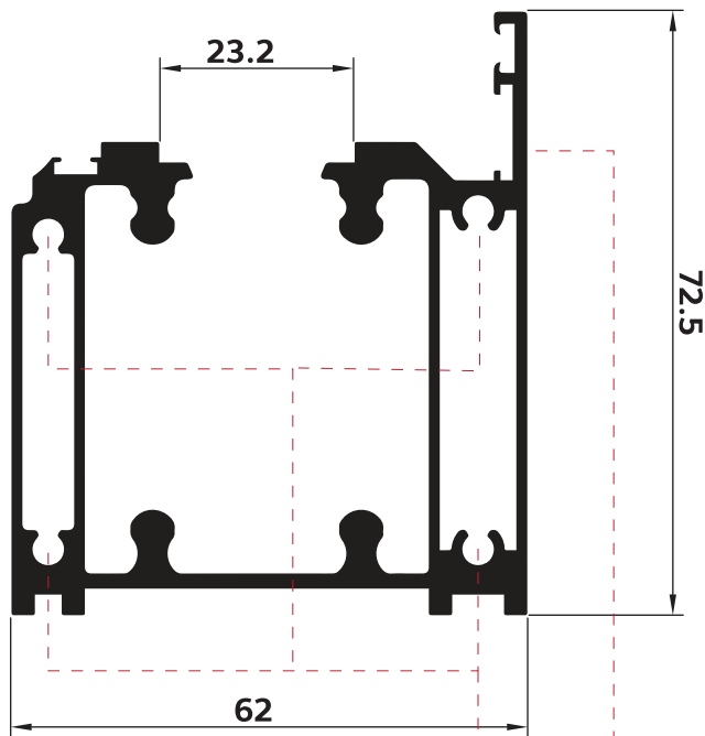
NEW P-204141 เฟรมบานพับ
