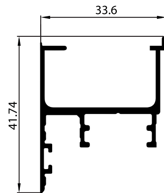
NEW P-174540 ชนกลางบานเปิด
