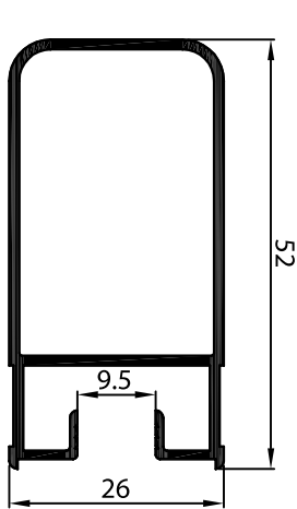
P-126779 เสาประตู ล็อค 1 จุด Single Lock 1.2 มม.
