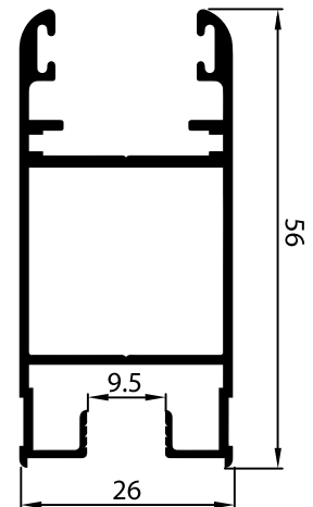
NEW P-124589 เสาประตู Multi-point Lock Euro
