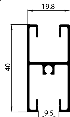
P-126787 ชนกลาง
