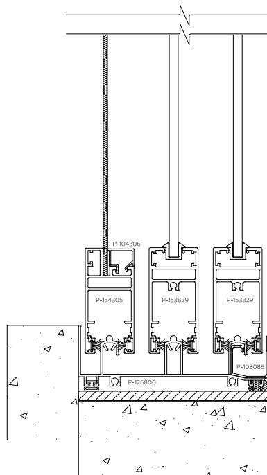
ประตูบานเลื่อนสลับ
