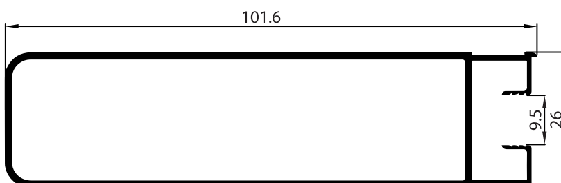
P-126782 เสาเลื่อน 1.2 มม.
