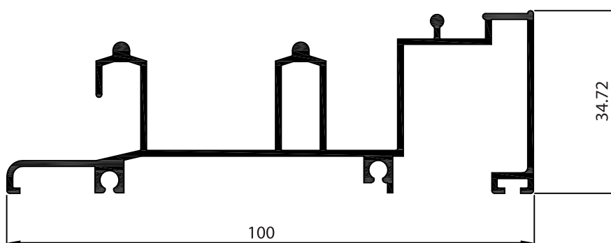
P-113512 เฟรม บาน-ล่าง 10 ซม. (กรณีเตี้ย)
