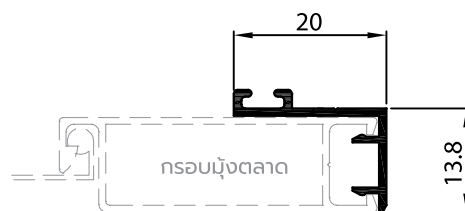
P-106797 ก้านแมลง (ใช้ร่วมกับมุ้งตาลาดทั่วไป)
