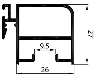
P-126782 เสาเลื่อน 1.2 มม.
