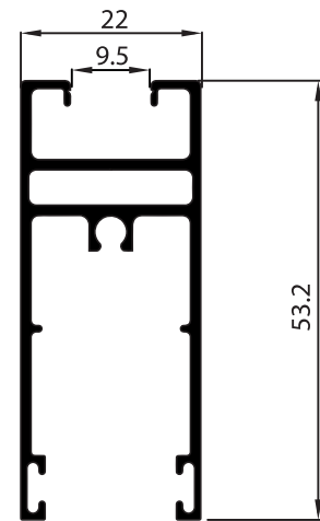
P-153624 ขวงบน-ล่าง 1.5 มม.
