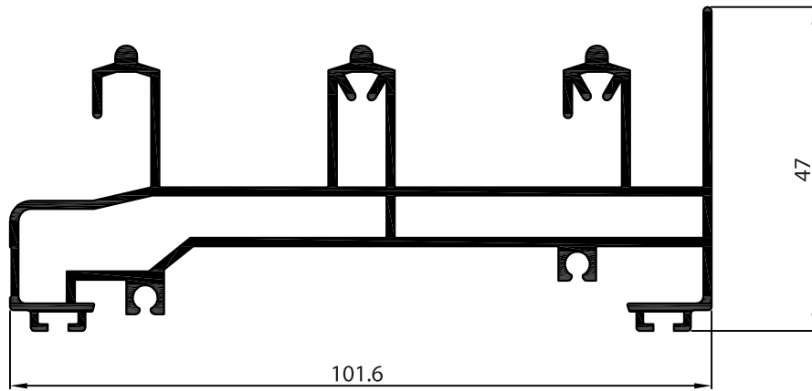
P-126804 เฟรม บาน-ล่าง 3 ราง
