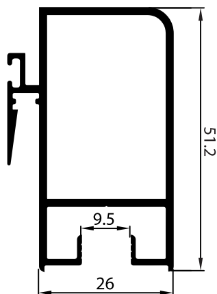
P-153622 เสาเลื่อน 1.5 มม.
