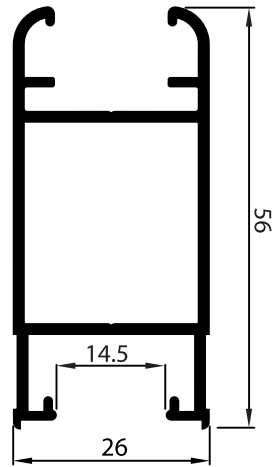
P-153628 เสาประตูร่องกว้าง 1.5 มม.
