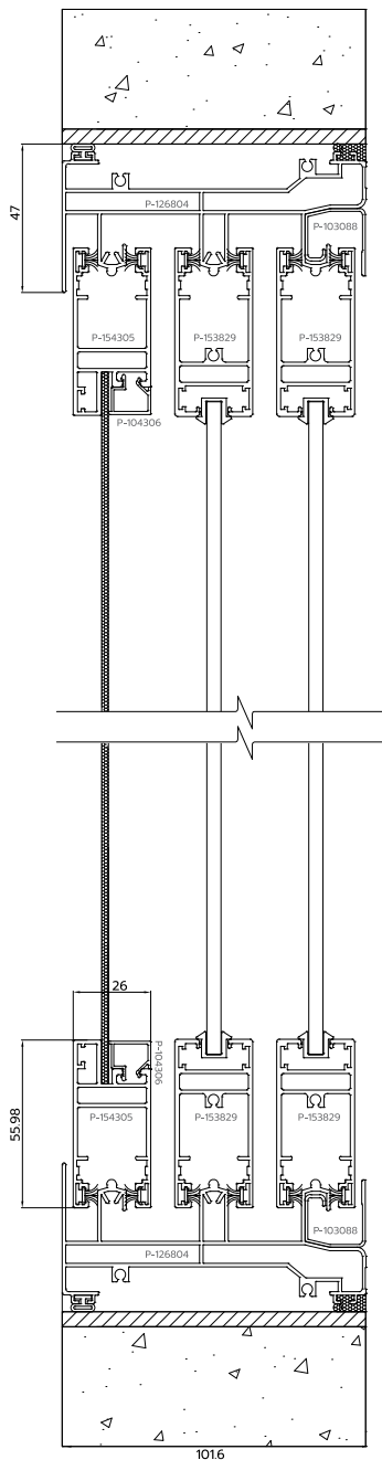
หน้าต่างบานเลื่อนสลับ
