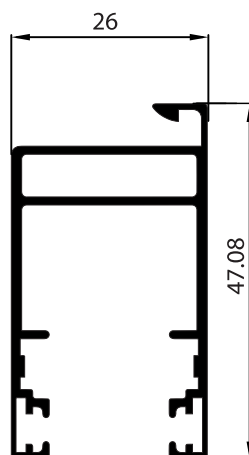
P-153872 กรอบมุ้ง บานเลื่อน 1.5 มม.
