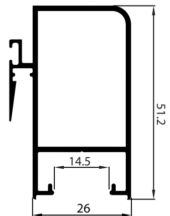
P-153623 เสาเลื่อนร่องกว้าง 1.5 มม.
