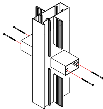
ภาพ Detail การเจาะและยึดของ แบ่งบานกับตัว P-123264 Adapter แบ่งบาน **กรณีไม่ใช้ สกัด ให้ใช้สกรูแบบเกลียวปลั๊ย M4 แทน
