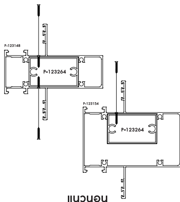
ภาพ Detail การเจาะและยึดของแบ่งบาน กับตัว P-123264 Adapter แบ่งบาน
