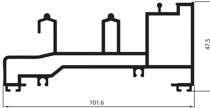
P-153620 เฟรม บาน-ล่าง 4 นิ้ว
