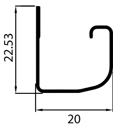
P-103088 ก้านตก (ใช้ร่วมกับเฟรมล่าง = ก้านตก) (ใช้ร่วมกับเฟรมบน = ก้านสาด)
