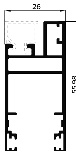
NEW P-154305 กรอบมุ้ง บานเลื่อน 1.5 มม.
