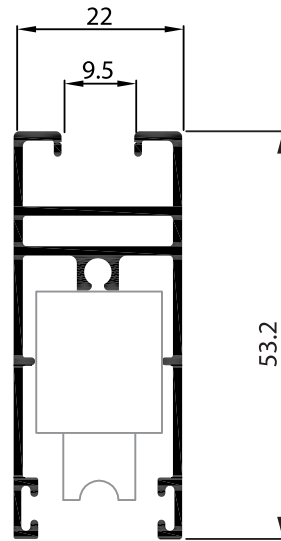
P-123167 ขวงบน-ล่าง (ล้อตลับร่องยู) *มี Hollow ป้องกันสกรูโดนกระชกแตก*
