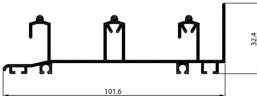
P-126800 เฟรม บาน-ล่าง 3 ราง (กรณีเตี้ย)
