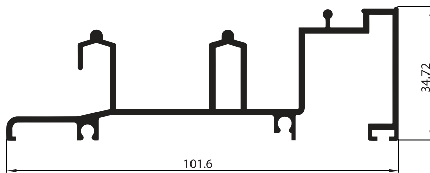
P-153621 เฟรม บาน-ล่าง 4 นิ้ว (กรณีเตี้ย)
