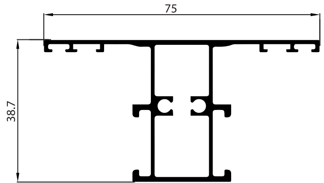
P-154061 แบ่งบานกระจก
