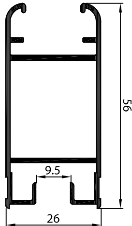
P-126780 เสาประตู ล็อคหลายจุด Multi-point Lock
