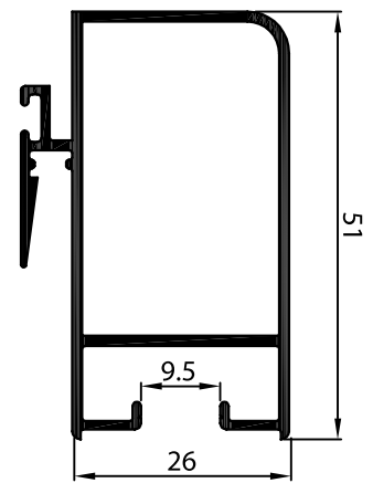
P-126781 เสาเลื่อนหน้าต่าง 1.2 มม.
