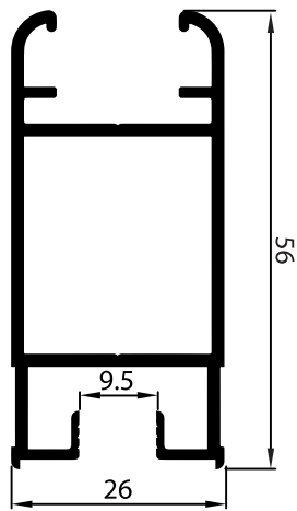
P-153627 เสาประตู 1.5 มม.
