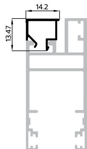
NEW P-104306 คิ้วมุ้งบานเลื่อน
